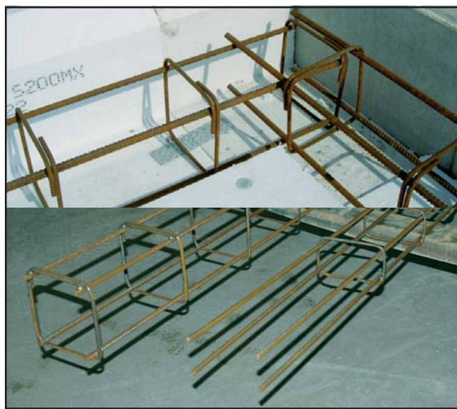
Färdigsvetsade armeringsbalkar
